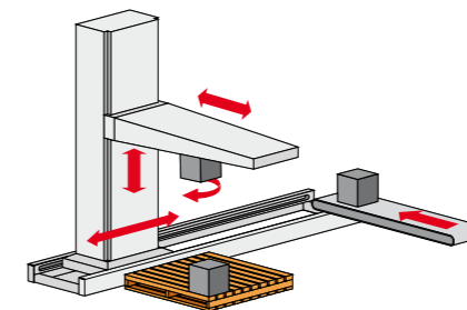
Der Produktablauf des meurer CM/MPR.
